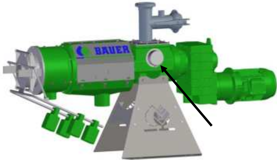
Abb. 16-1 Füllstandssensor
