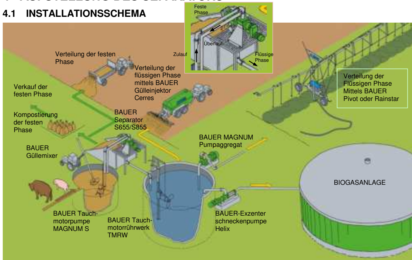
Abb. 4-1 Installationsschema
